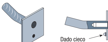
Piastra Zancata PZ2
