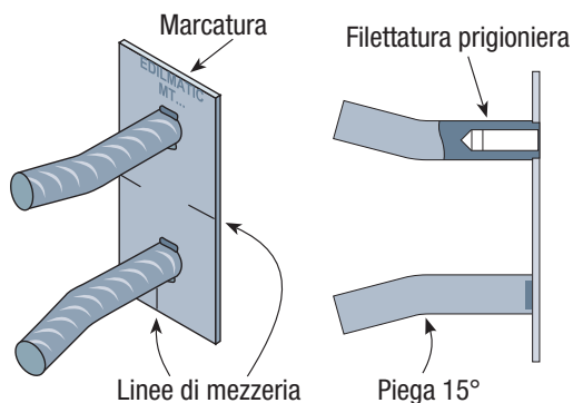
Piastra Zancata PZ4-6-9
